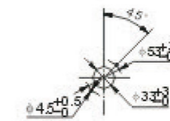
B型手柄面板开孔尺寸
